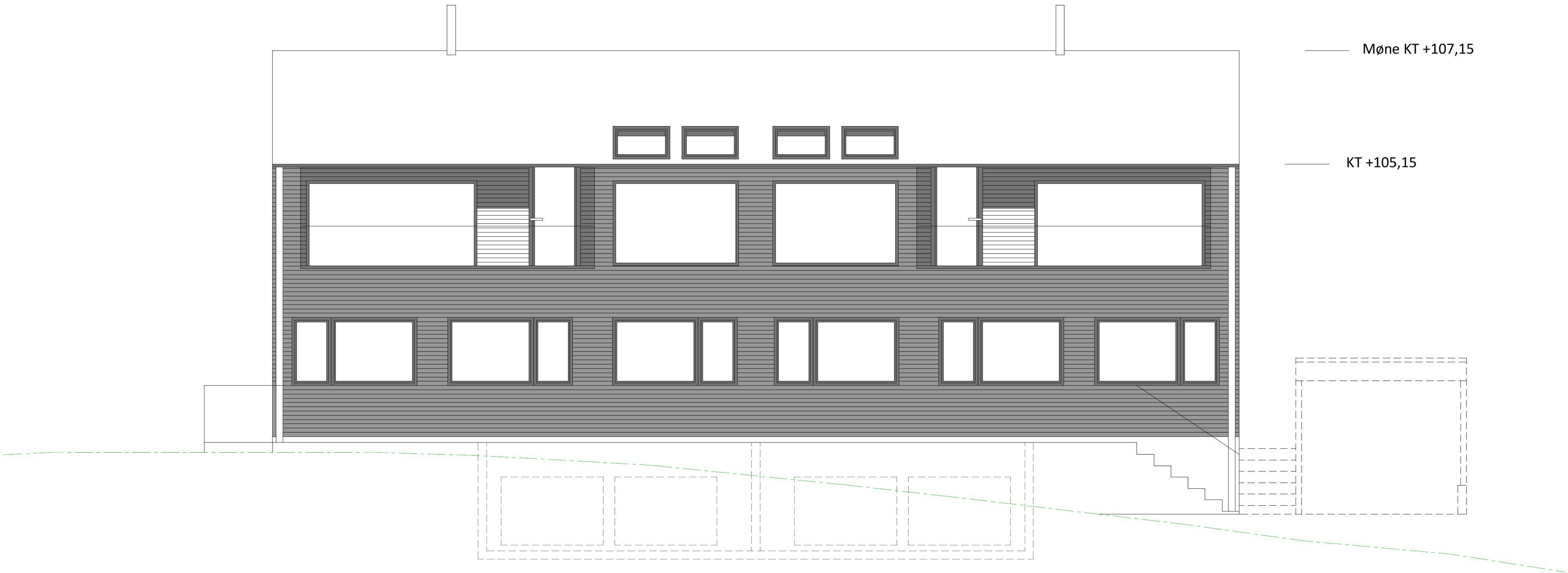
Fasade nordøst
